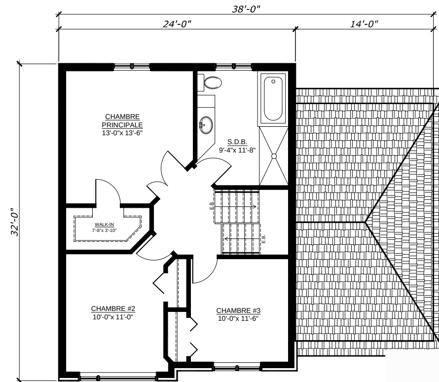
PLAN DE L'ÉTAGE SUPERFICIE HABITABLE ÉTAGE: 756 P 2 SUPERFICIE HABITABLE TOTALE: 1512 P 2
